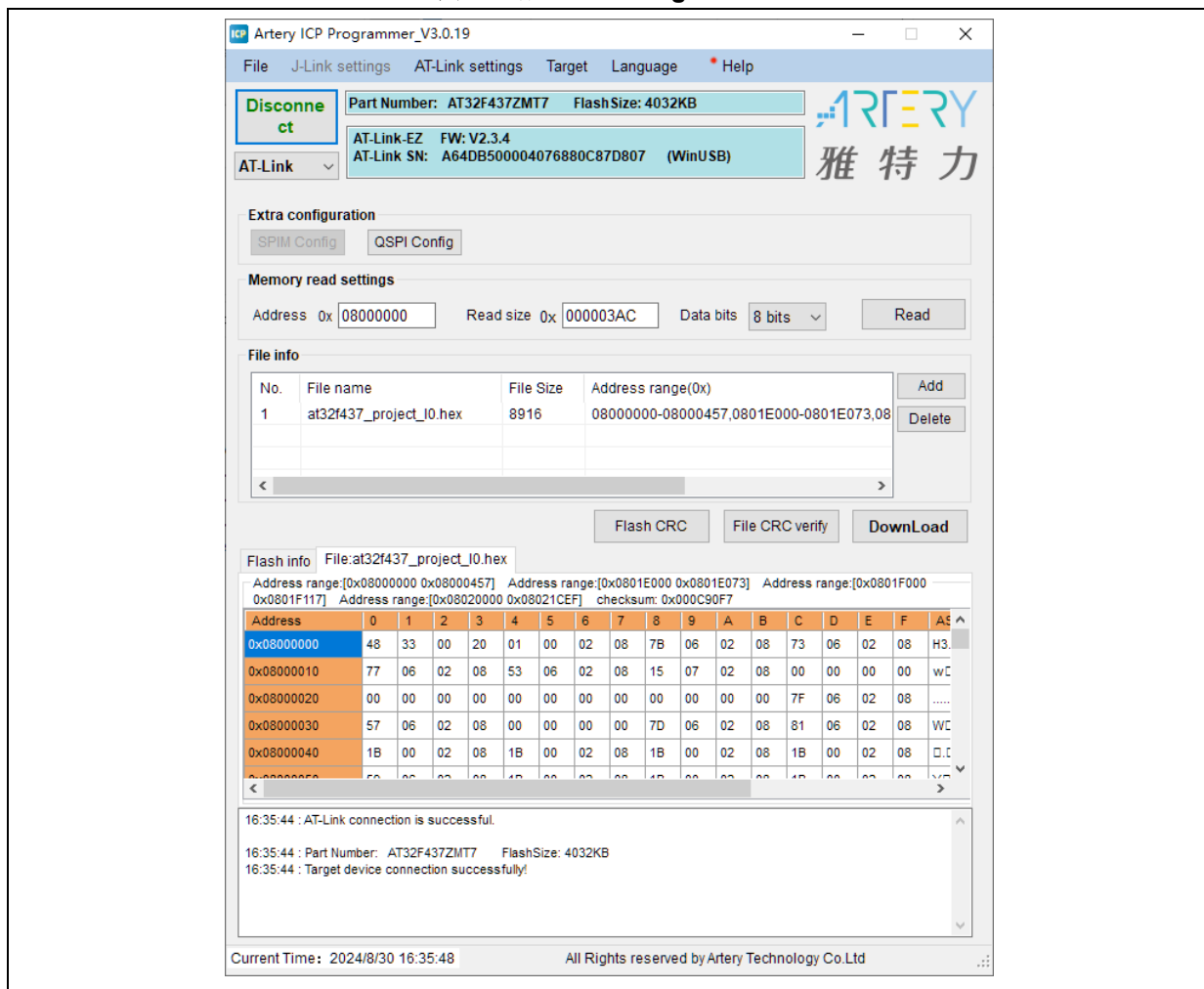
图 25. 配置 ICP Programmer
