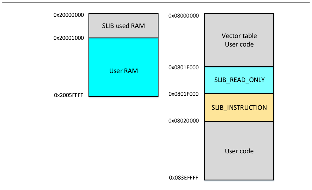
图 15. 范例程序的主闪存映像及 RAM 分区
