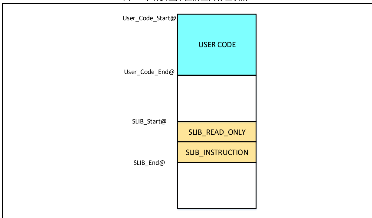
图 1. 带有安全库区的主闪存区映射
