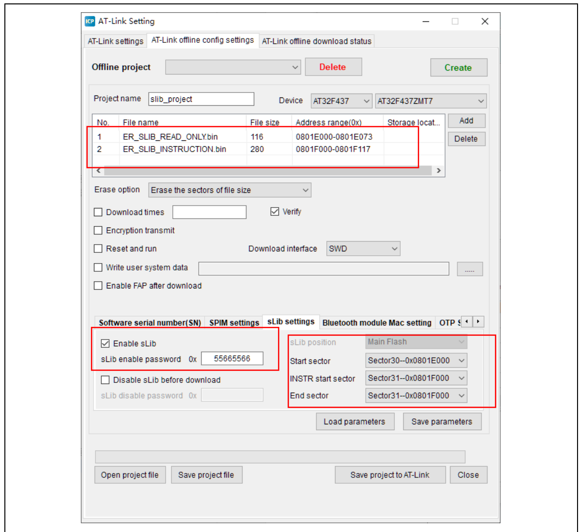
图 50. AT-Link 离线烧录到 MCU
