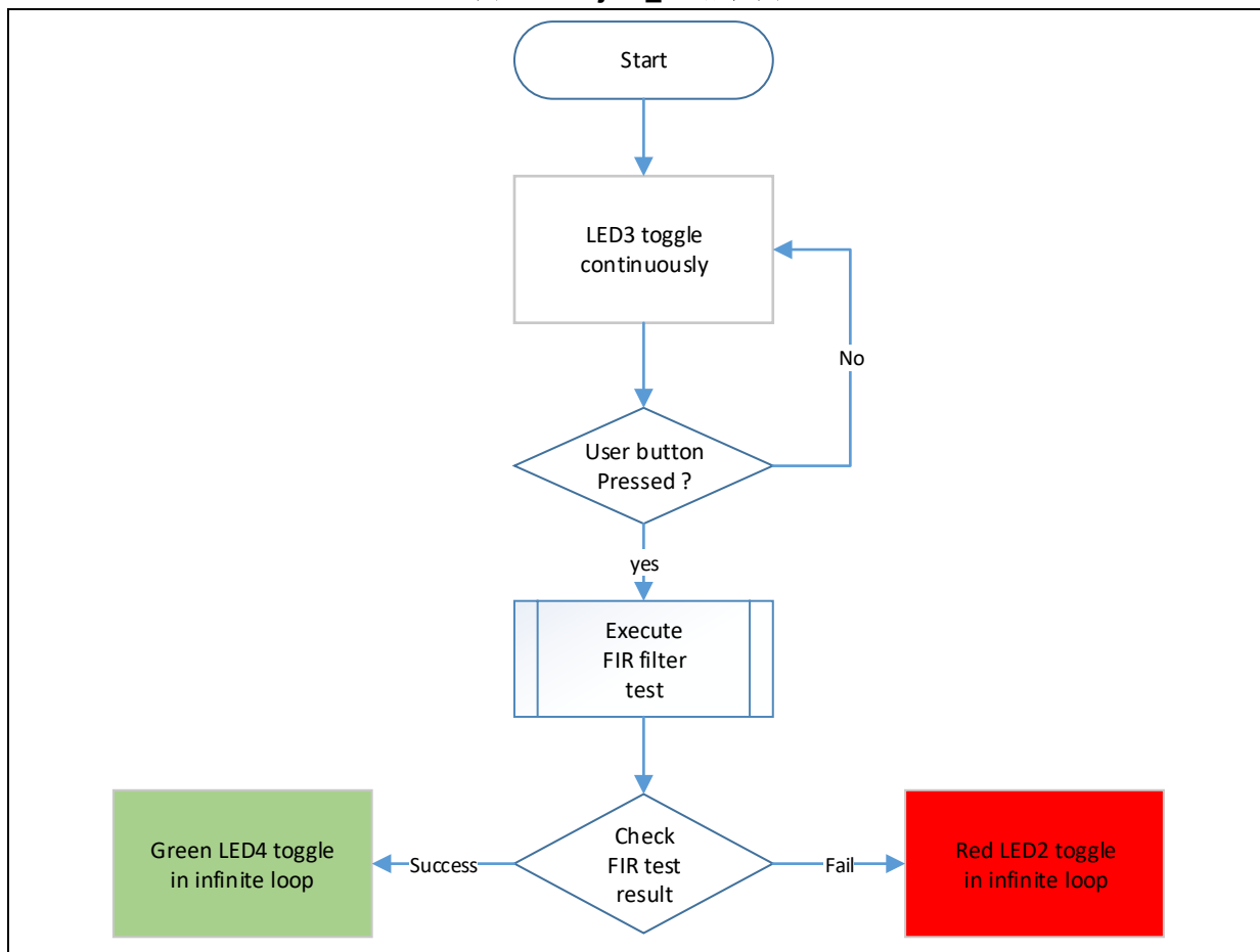
图 40. Project_L1 流程图
