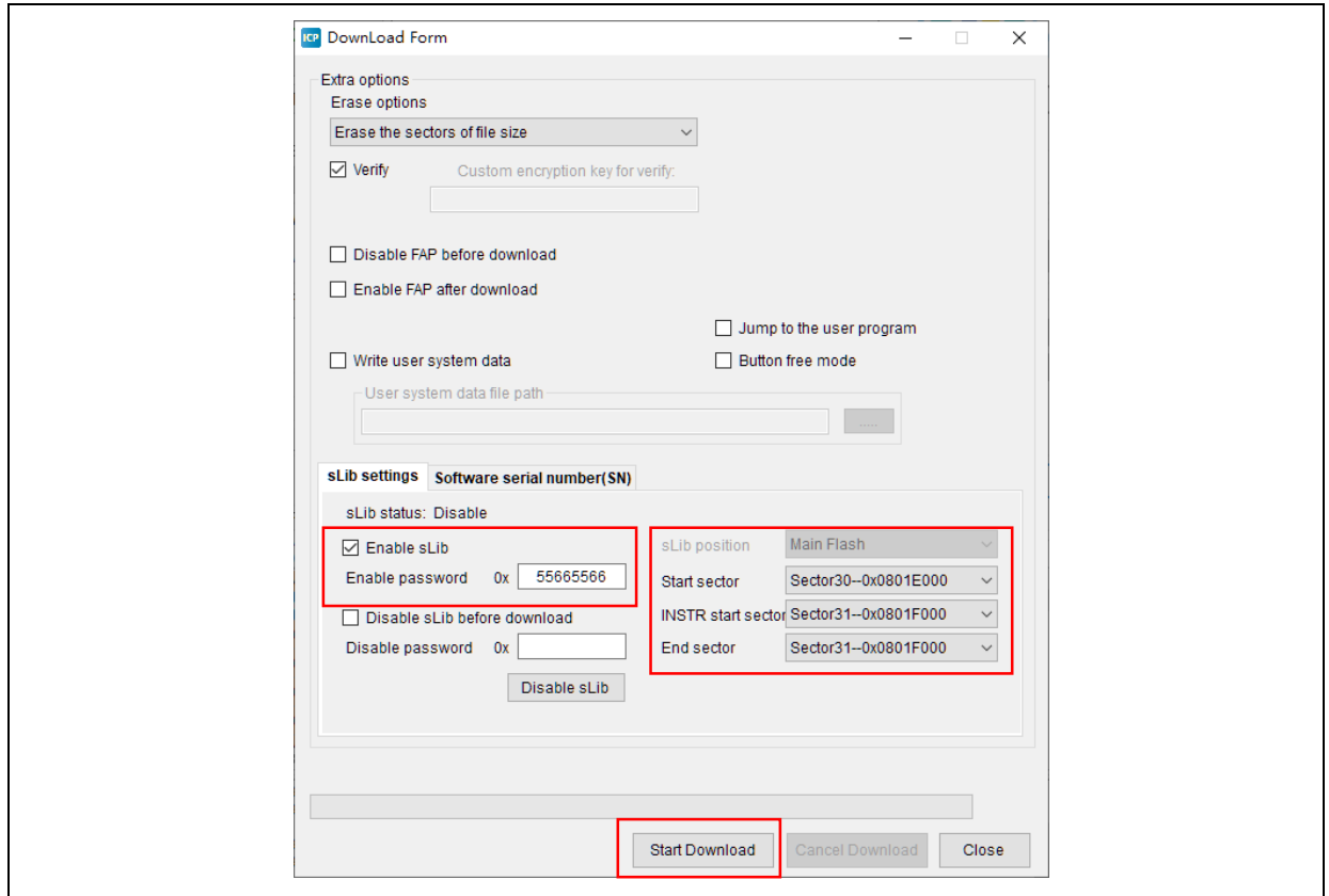
图 26. 设置下载选项参数
